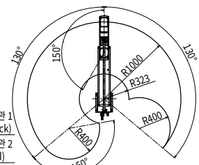
오른손잡이 시스템의 동작 범위
