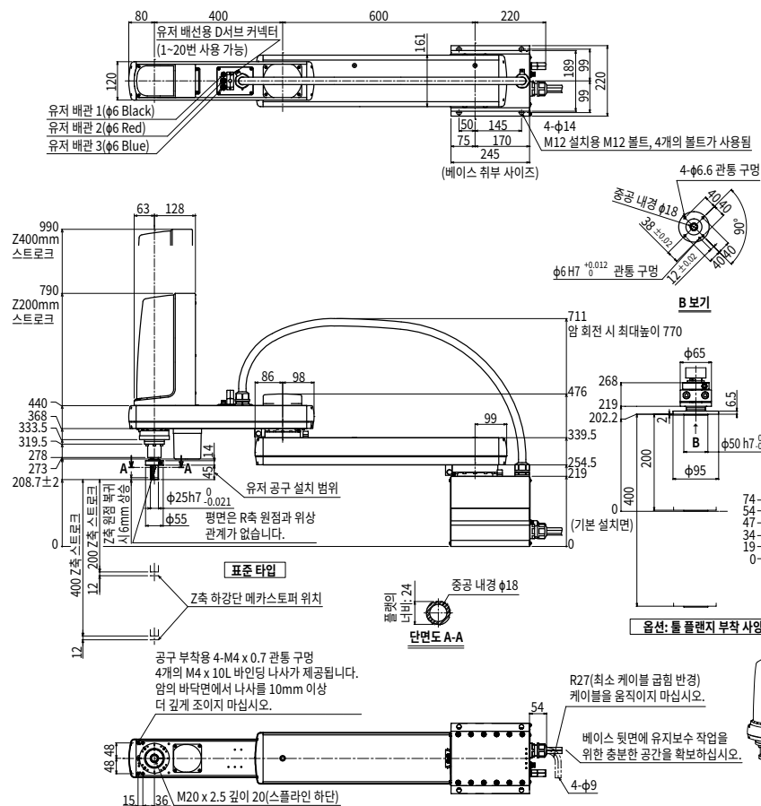
YK1000XG Z200mm 스트로크 사양
