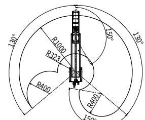
원손잡이 시스템의 동작 범위
